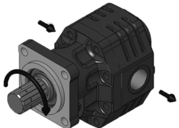
Right Rotation
