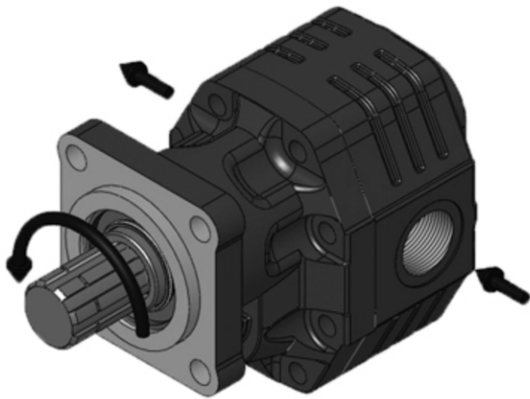
Left Rotation
